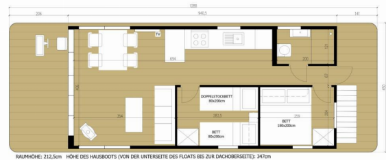
RAUMHÖHE: 212,5cm HÖHE DES HAUSBOOTS (VON DER UNTERSEITE DES FLOATS BIS ZUR DACHBEREICHE): 347cm
